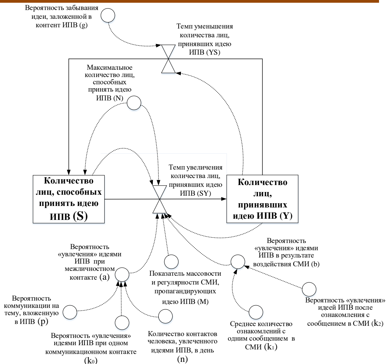
Рис. 1. Системно-динамическая модель влияния ИПВ на массовое сознание Fig. 1. System dynamics model of the impact of IPV on mass consciousness
