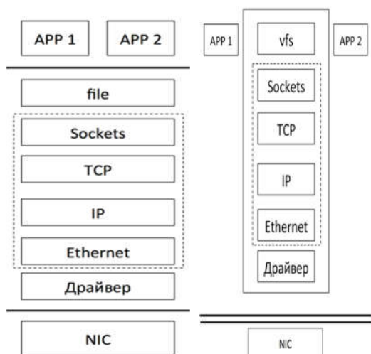
Рис. 2. Монолитный стек в пространстве пользователя
