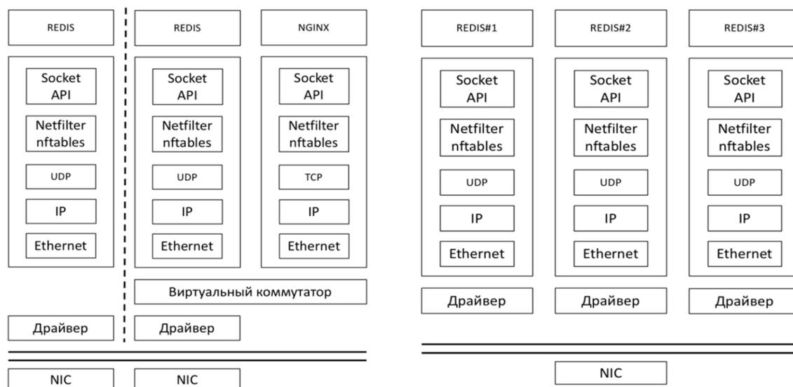
Рис. 5: Хранилище «ключ - значение»
