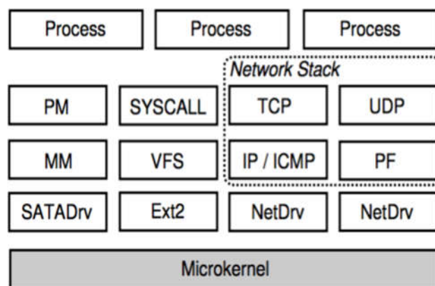
Рис. 3. Сетевая подсистема NewtOS
